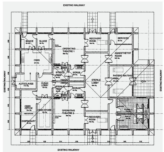
Grundriss für den neuen Operationssaal im Spital Phalombe
